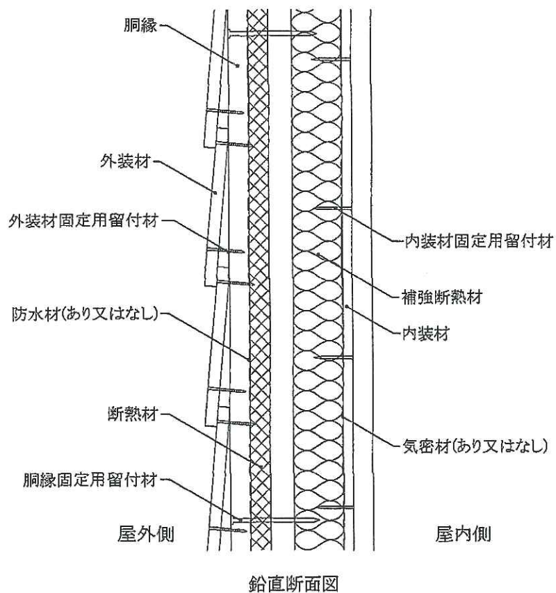
図6 構造説明図
