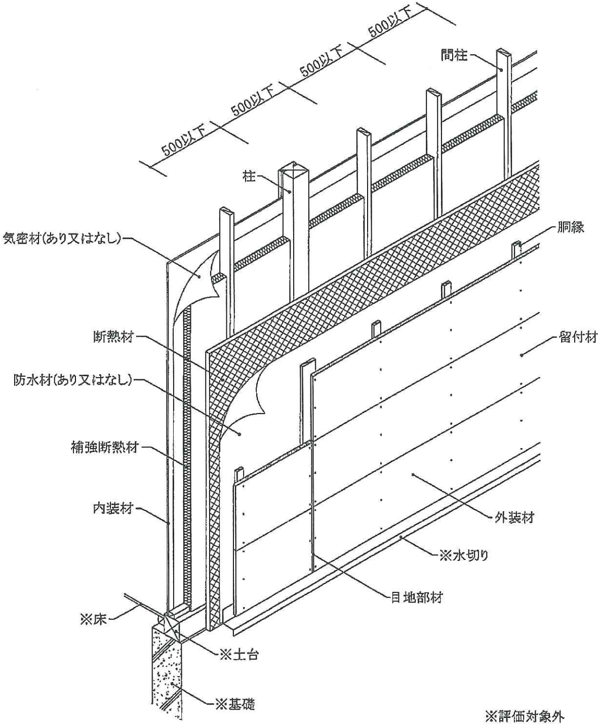
透視図
