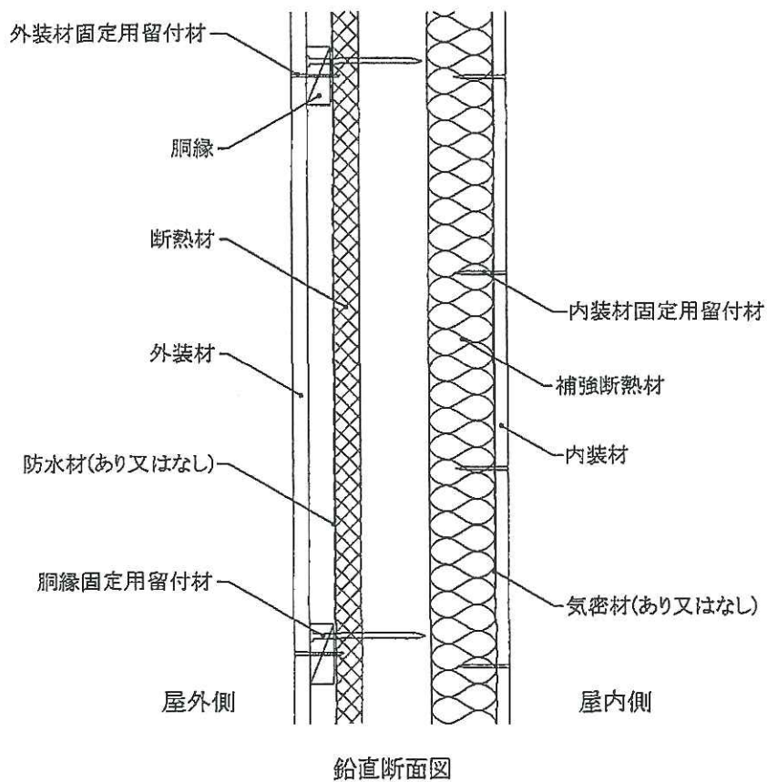
図 1 6 構造説明図
