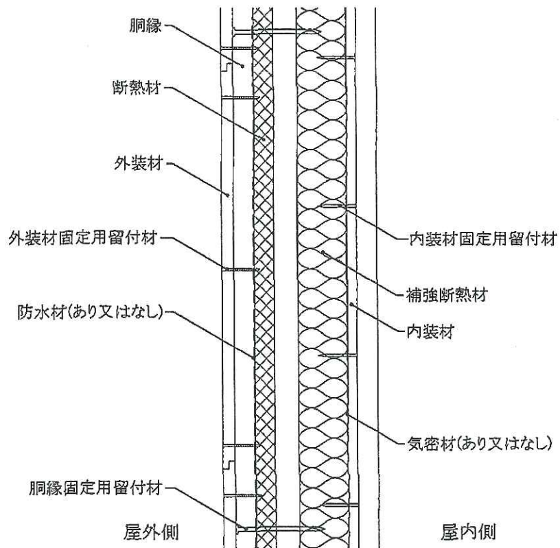
図 2 構造説明図
