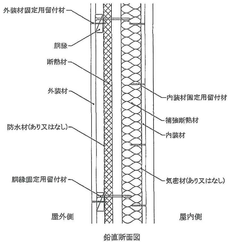
図 10 構造説明図
