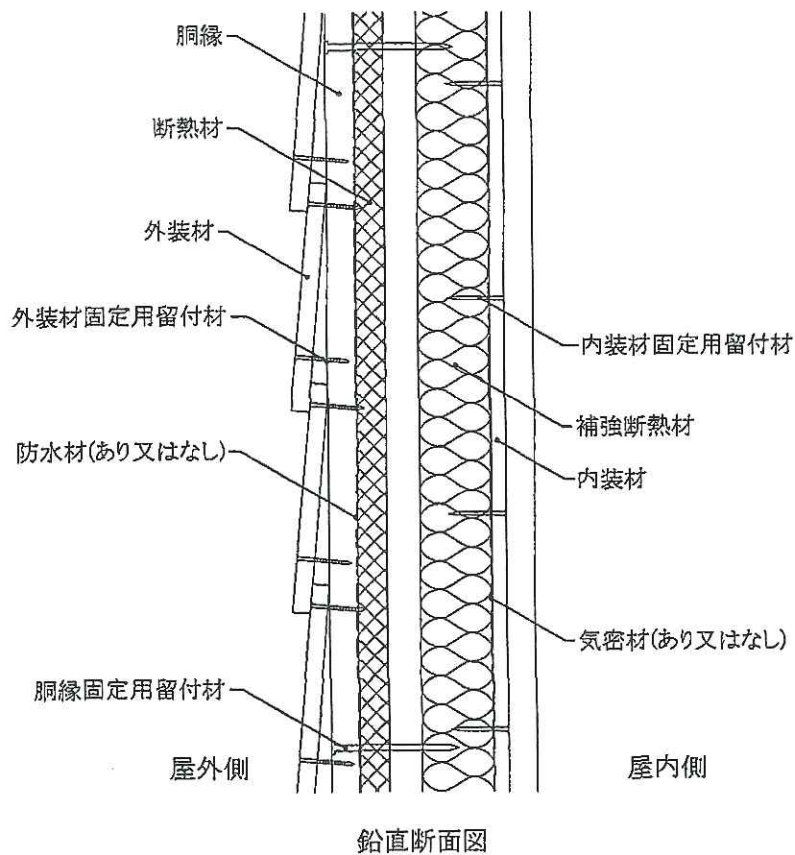
図 1 2 構造説明図
