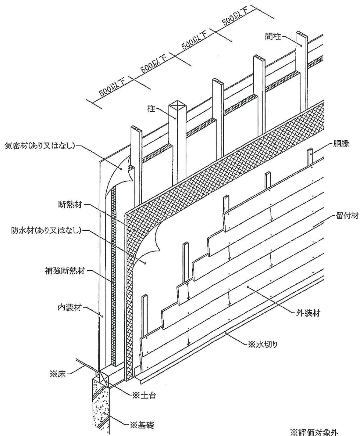
透視図
