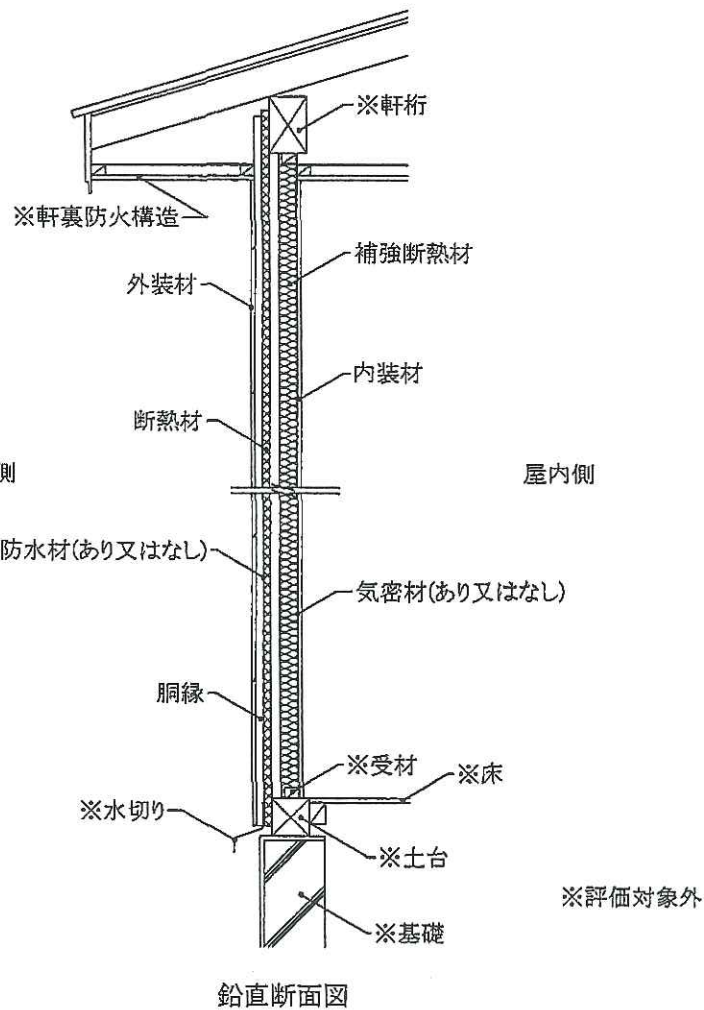
図 2 2 施工図
