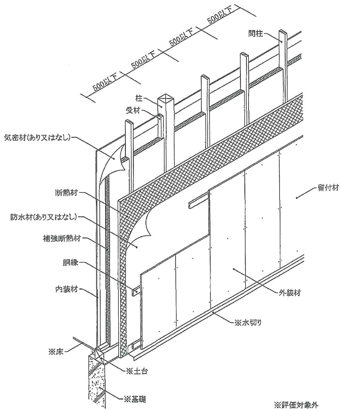
透視図
