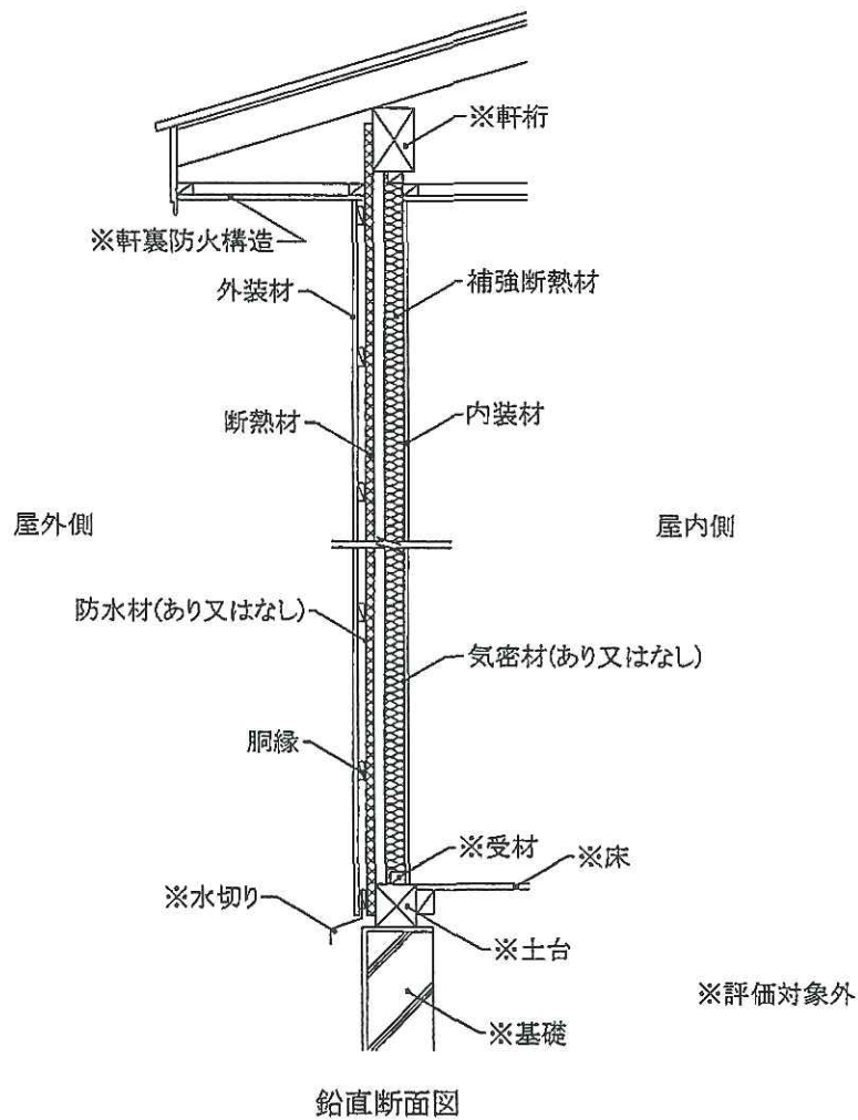
図 2 3 施工図
