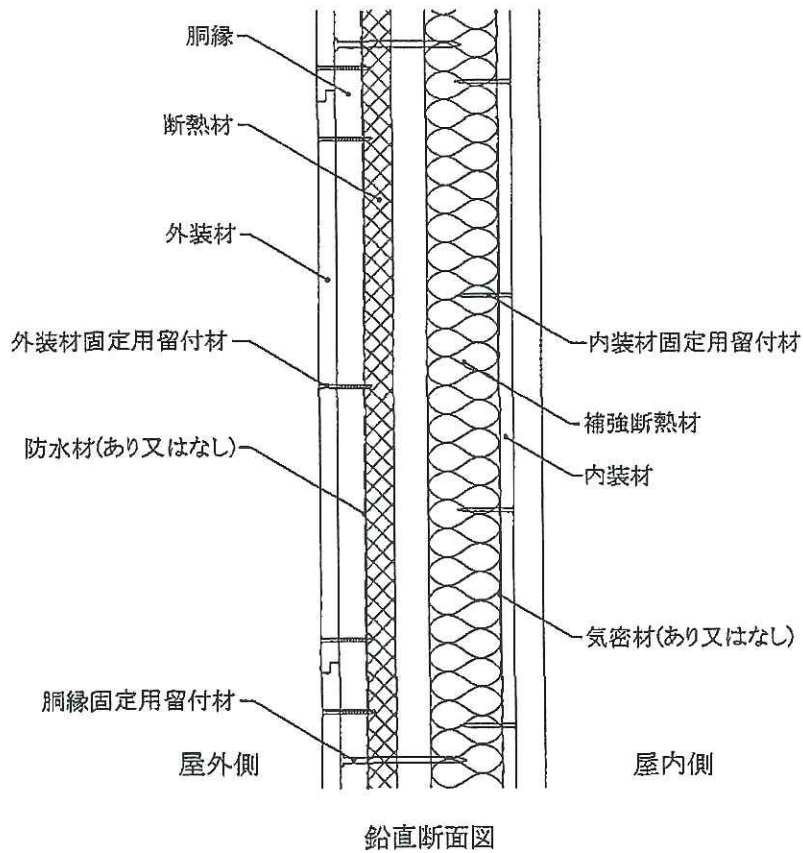
図8 構造説明図
