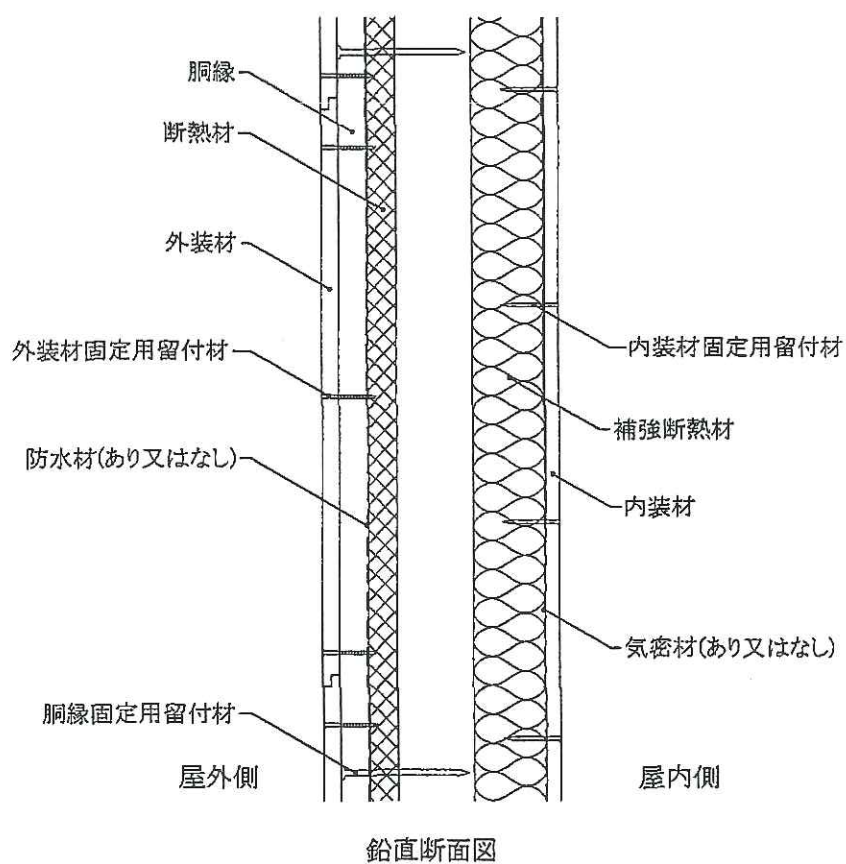
図 1 4 構造説明図
