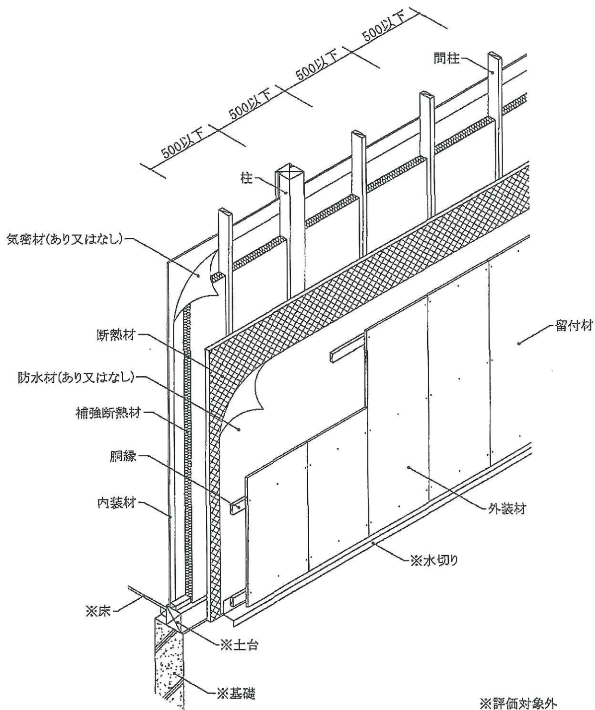
透視図
