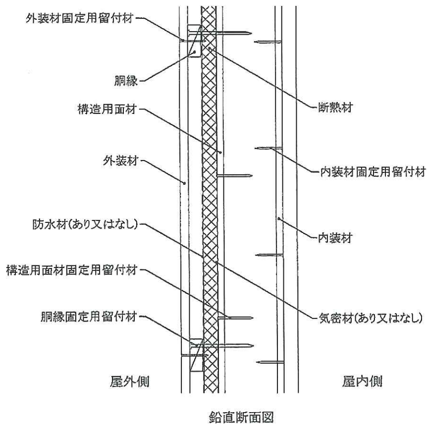
図10 構造説明図
