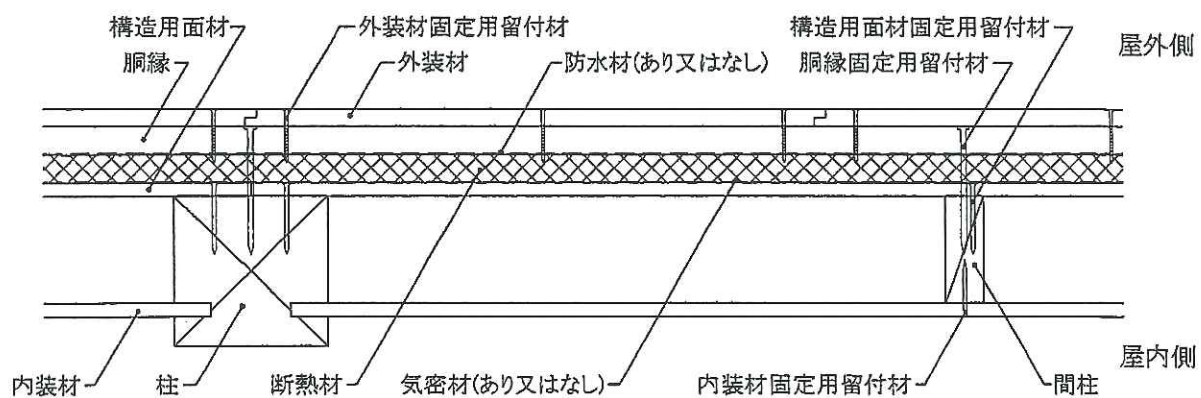
水平断面図
