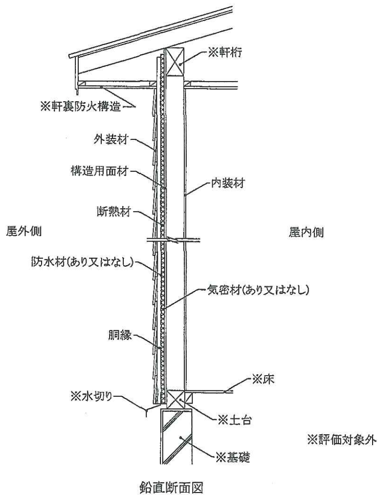
図 3 0 施工図
