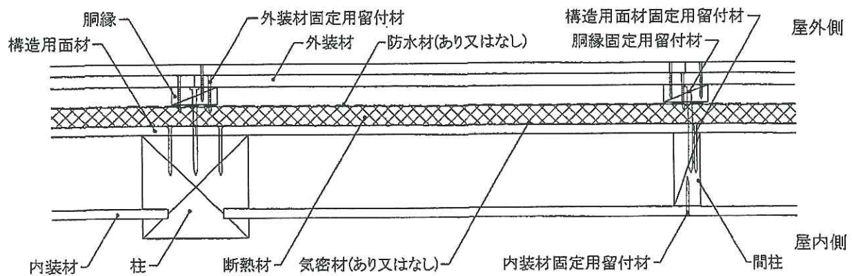
水平断面図
