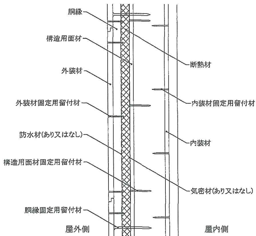
図2 構造説明図
