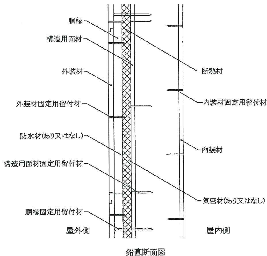
図 1 4 構造説明図
