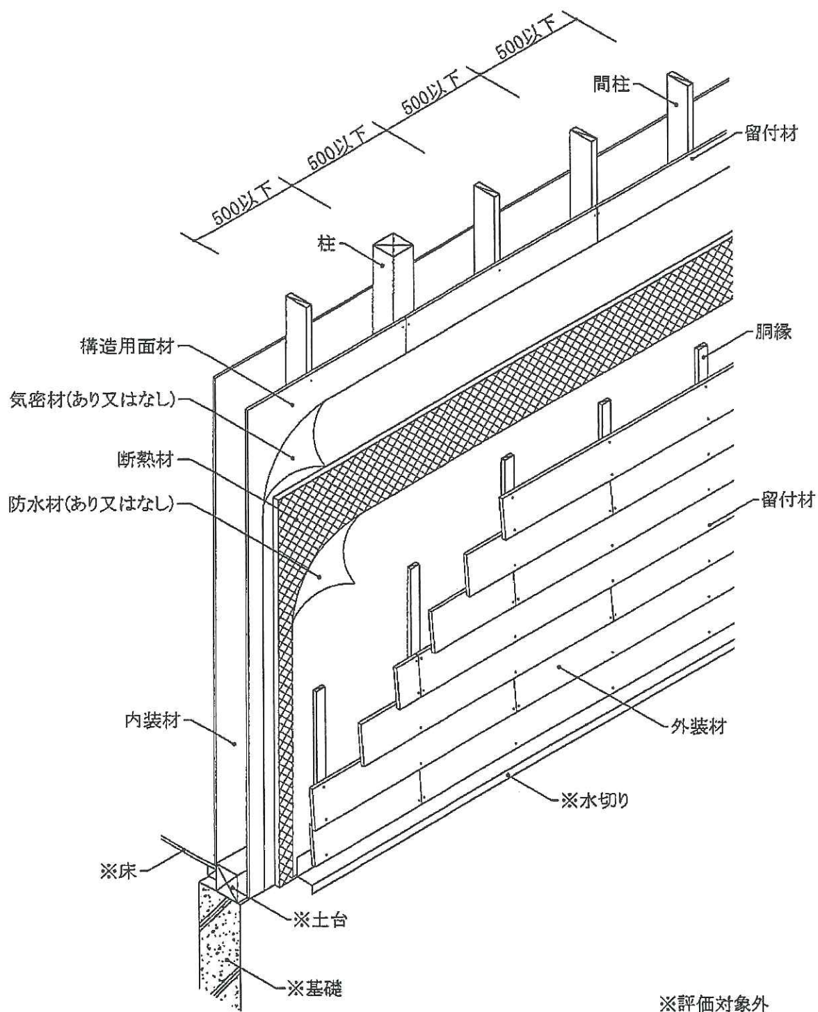
透視圖
