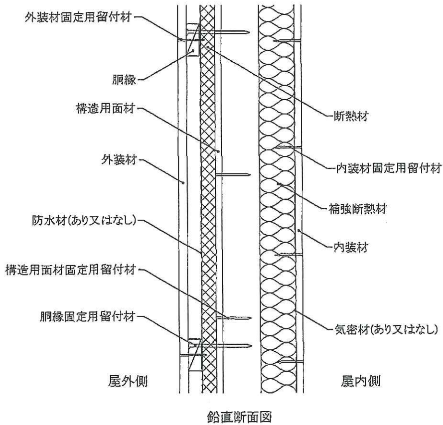
図 1 6 構造説明図
