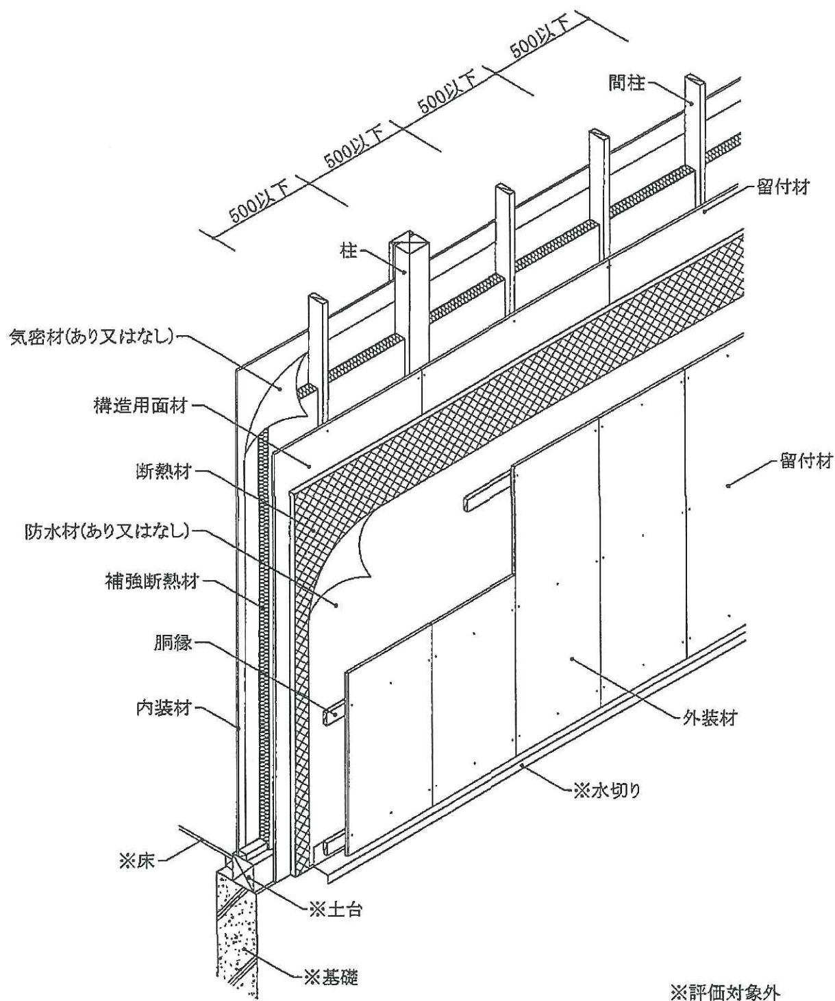
透視図
