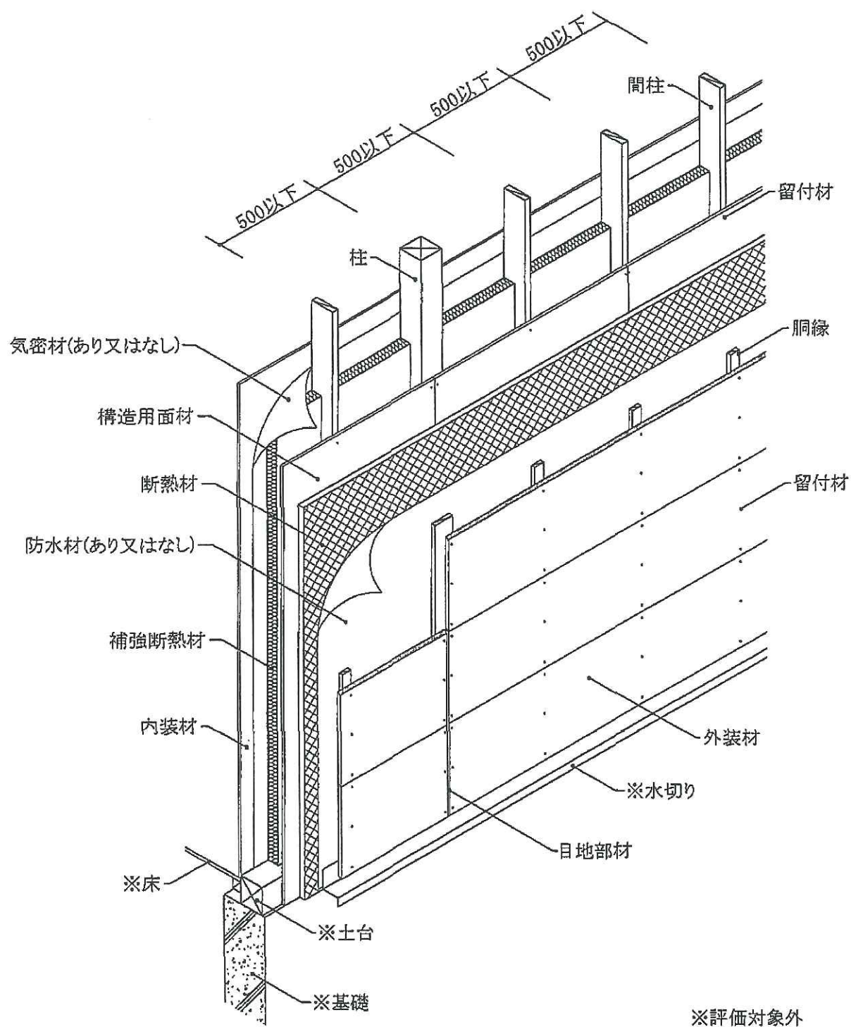
透視図
