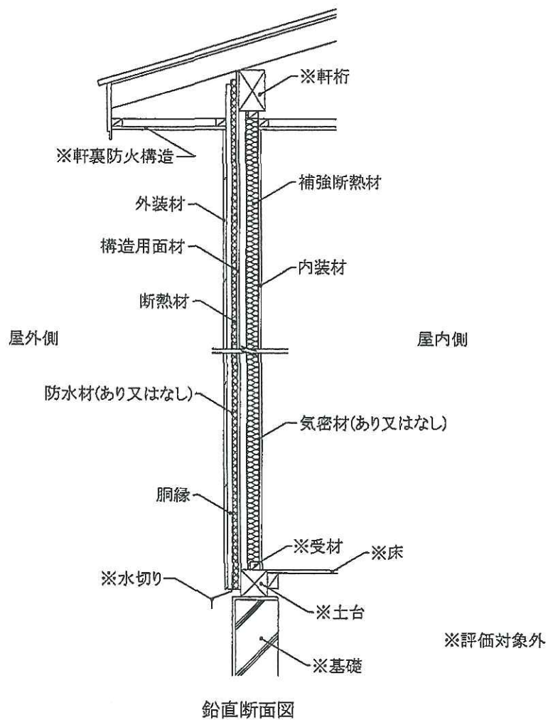
図 2 5 施工図
