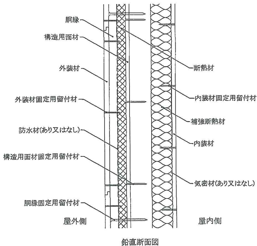
図 1 4 構造説明図
