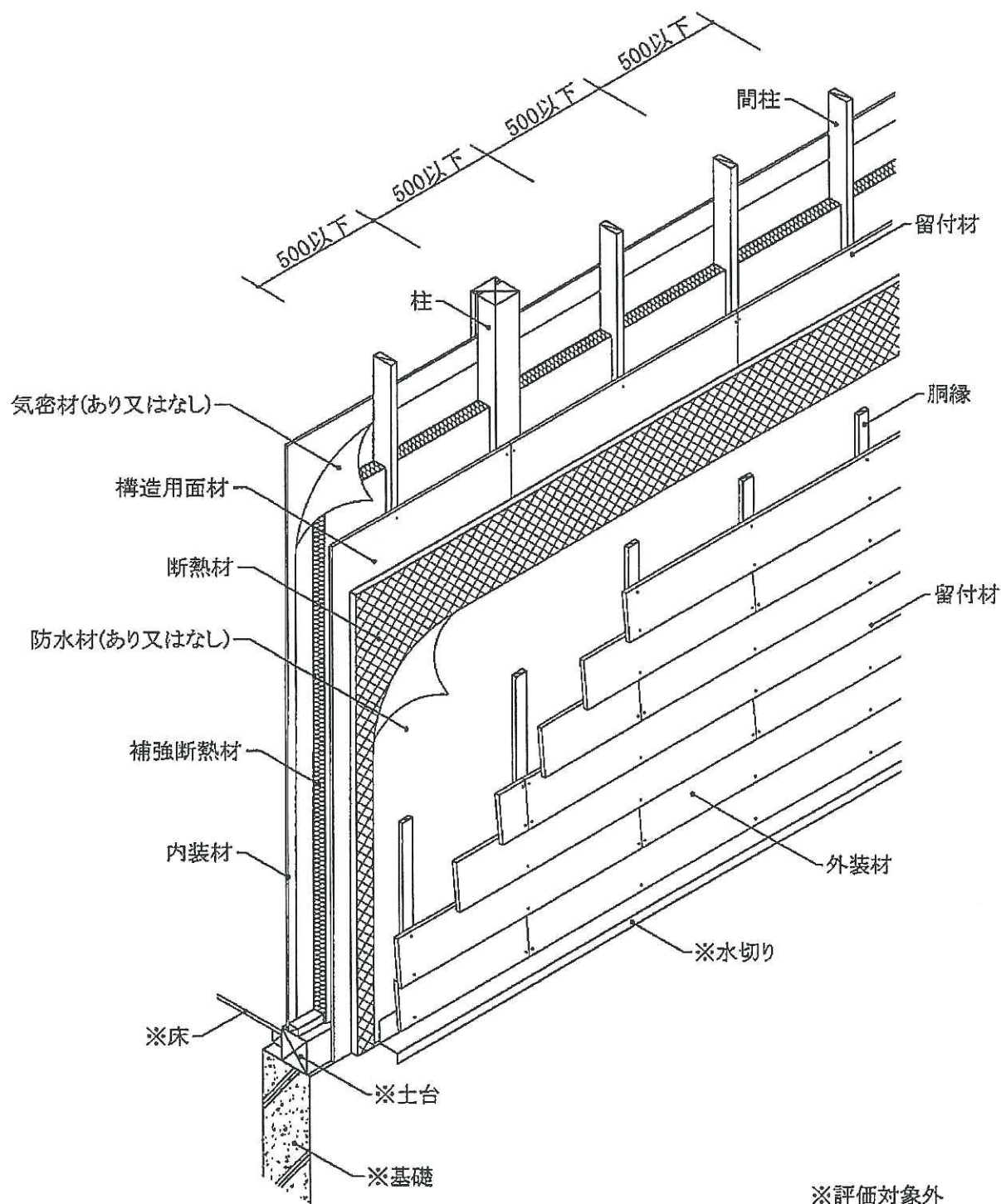
透視図
