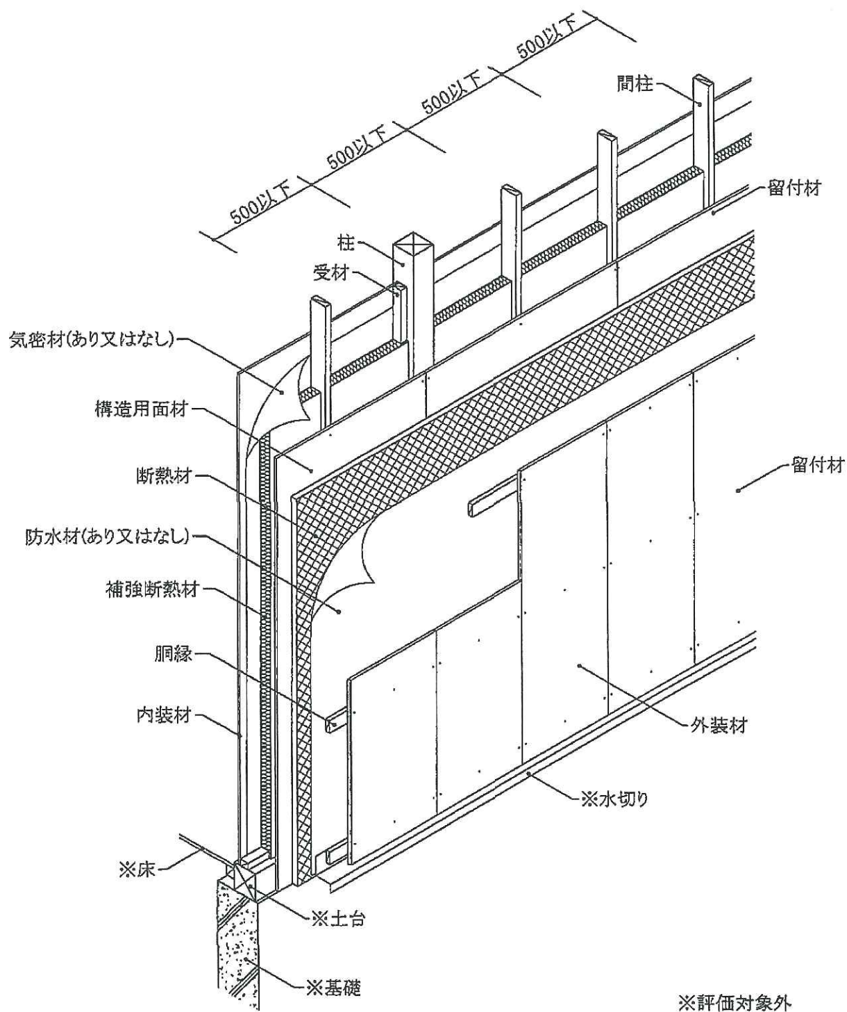
透視図
