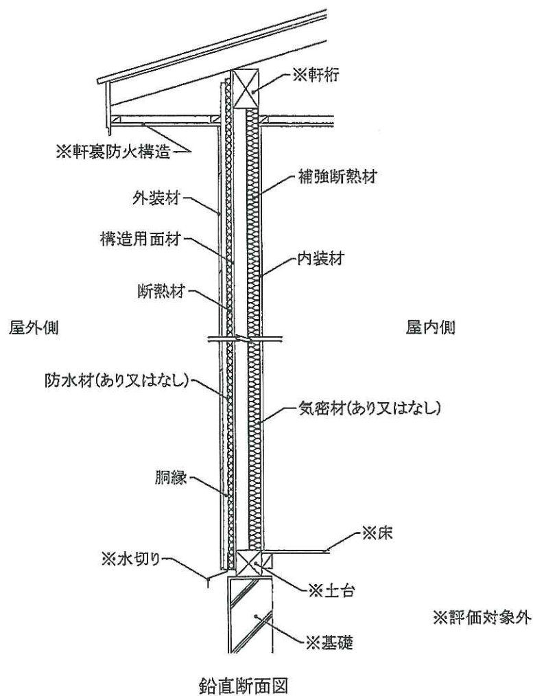
図 2 8 施工図
