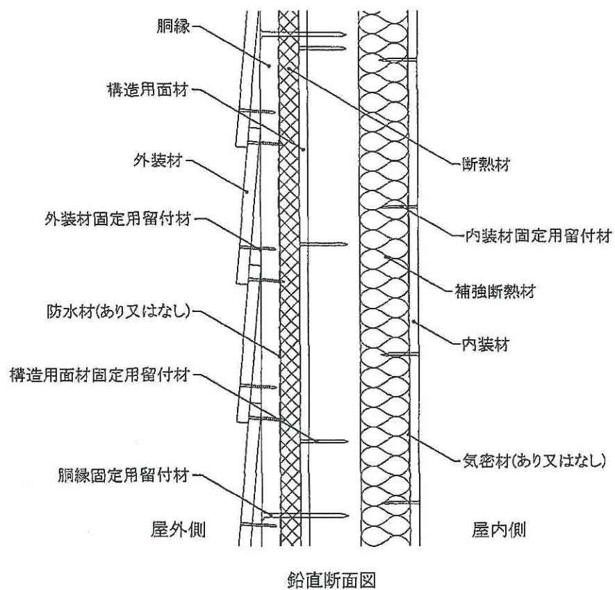
図 1 8 構造説明図
