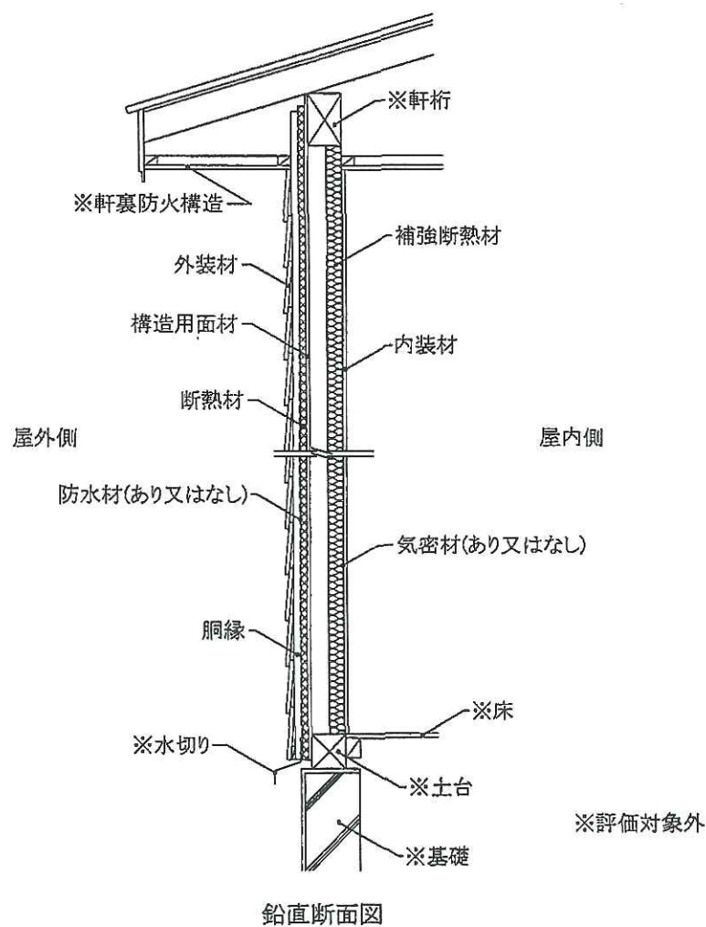
図30 施工図
