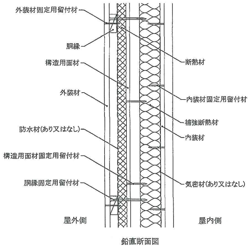
図 1 0 構造説明図
