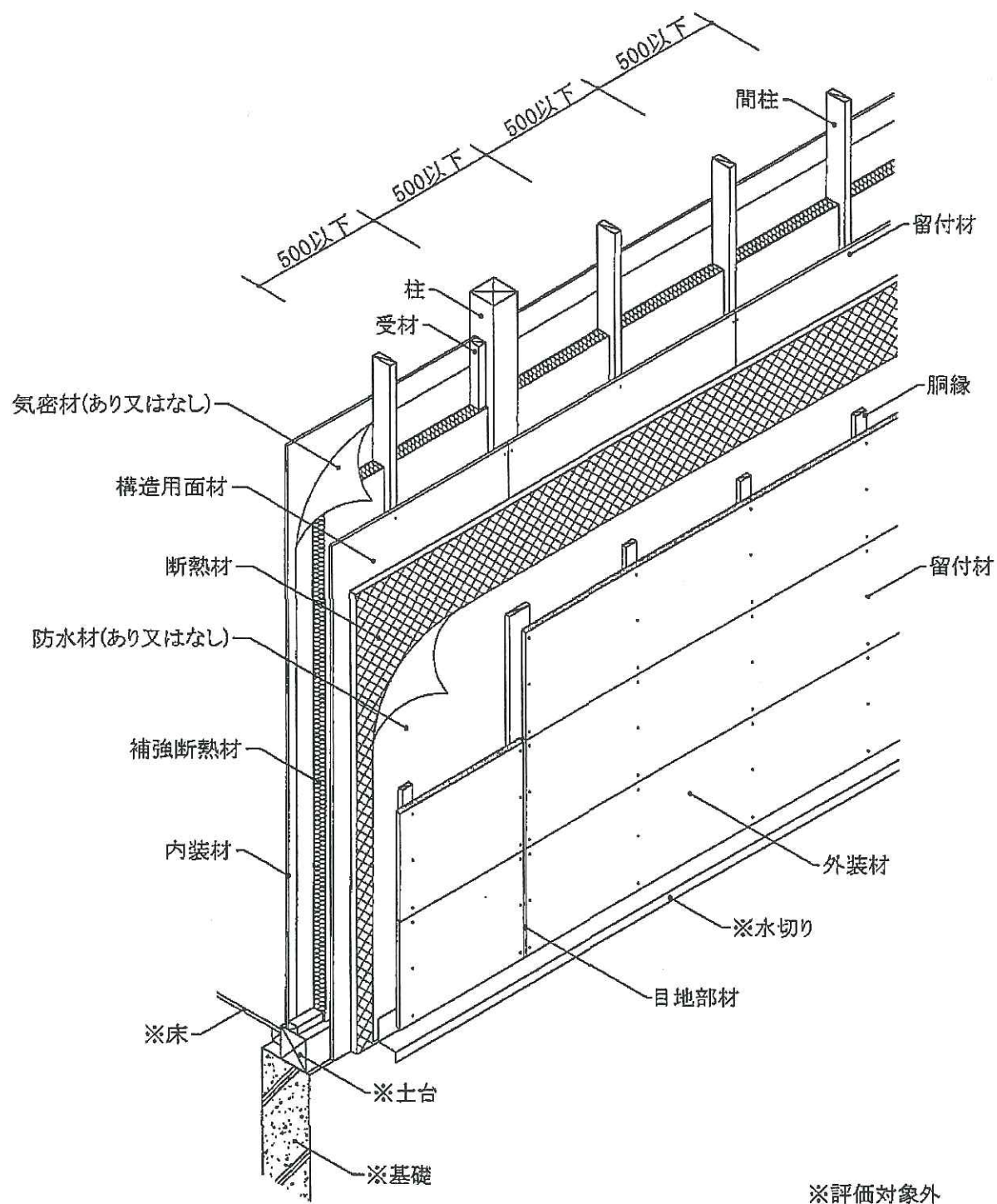
透視図
