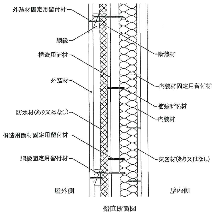
図4 構造説明図
