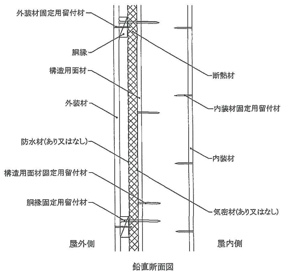
図 1 6 構造説明図
