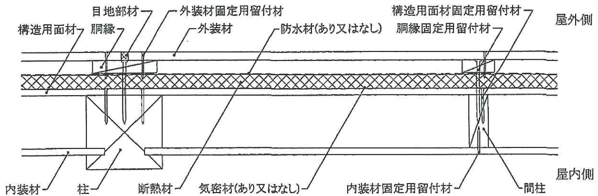
水平断面図
