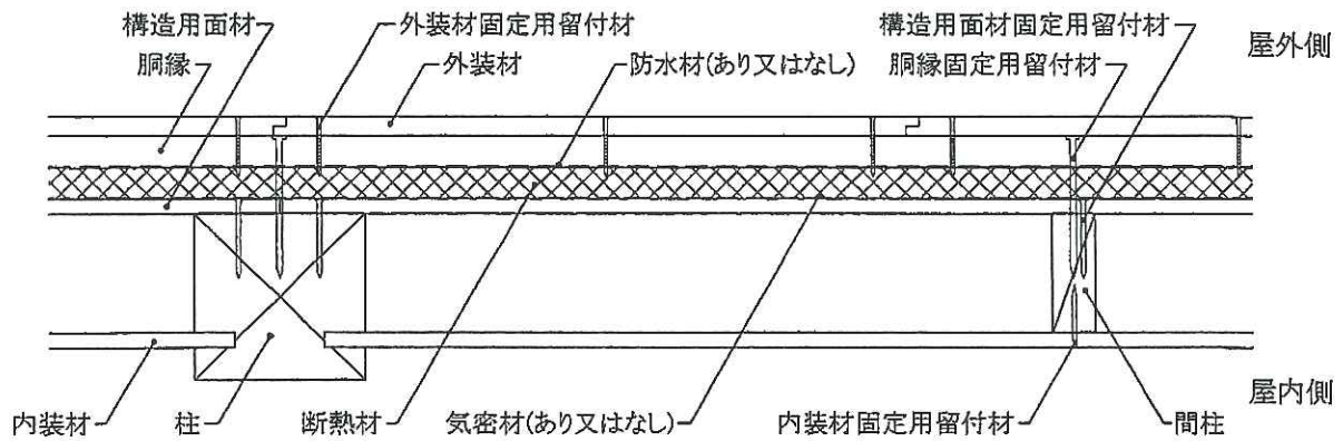
水平断面図
