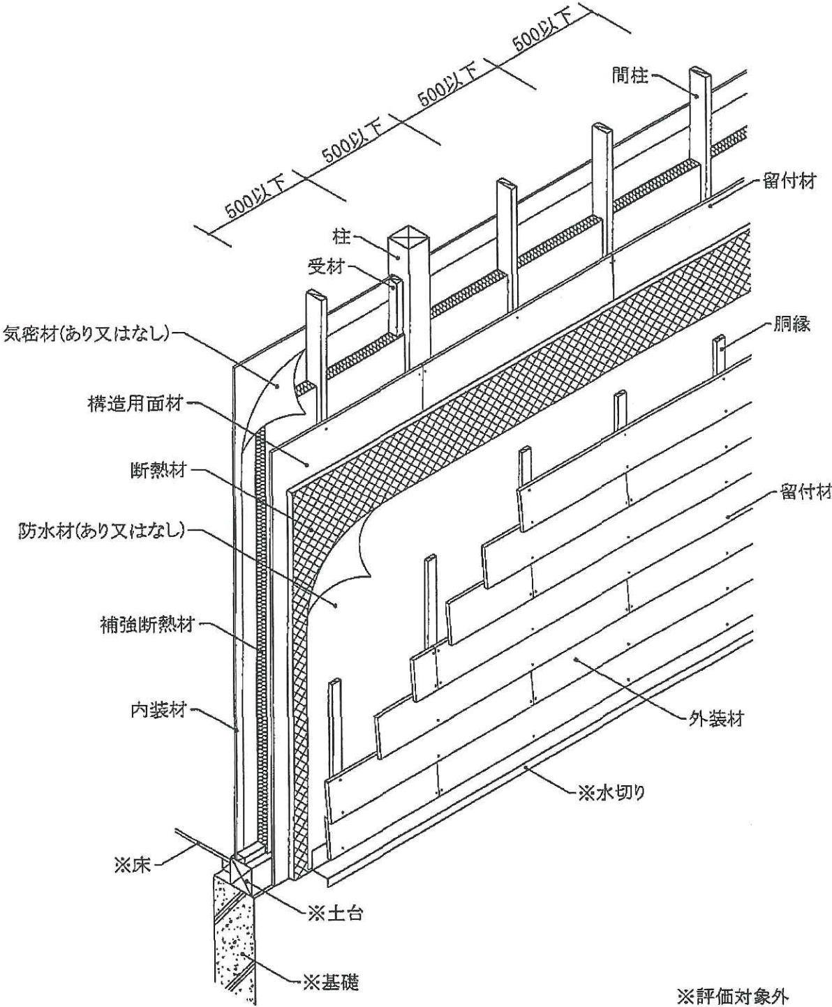
透視図
