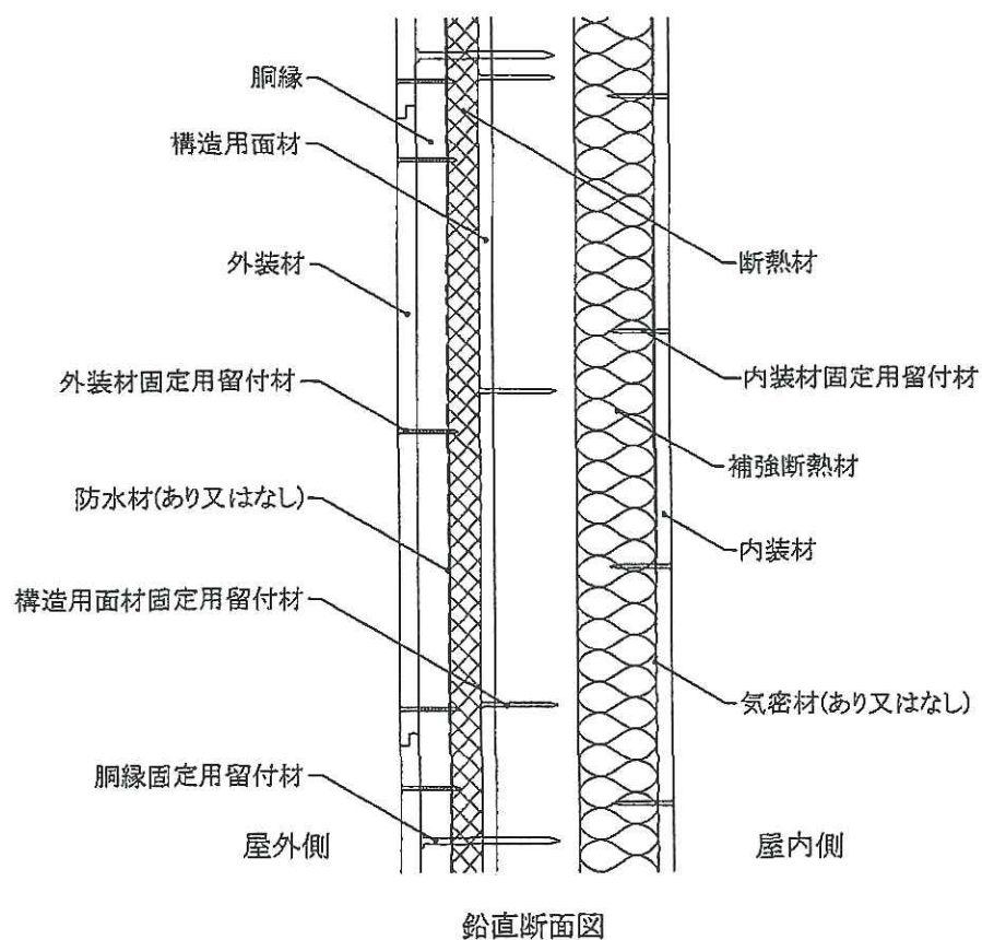
図 1 4 構造説明図
