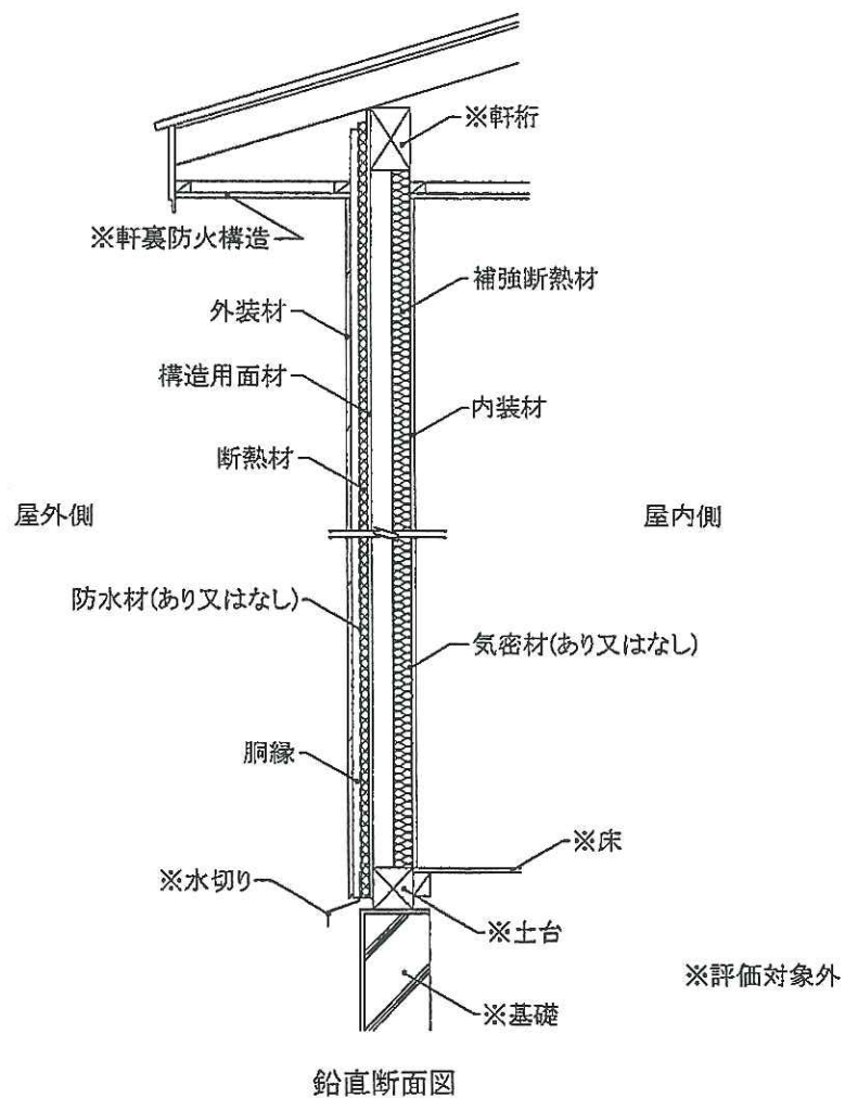
図 2 8 施工図
