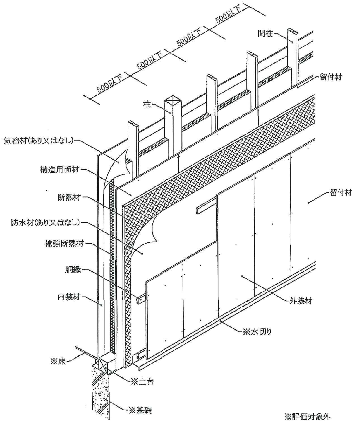
透視図
