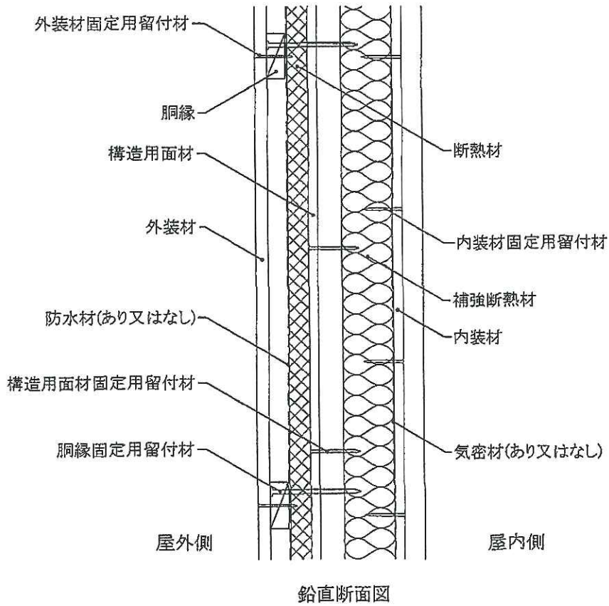
図 1 0 構造説明図
