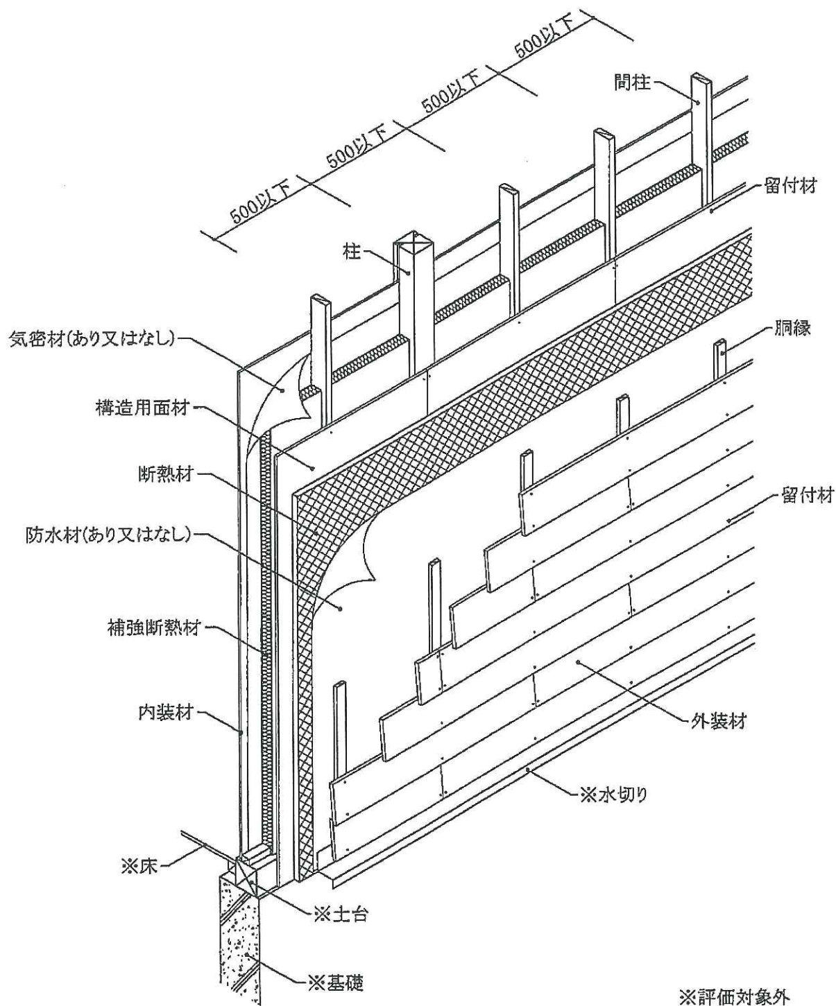
透視図
