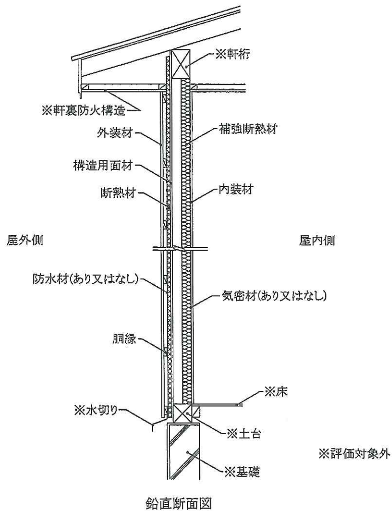
図 2 9 施工図
