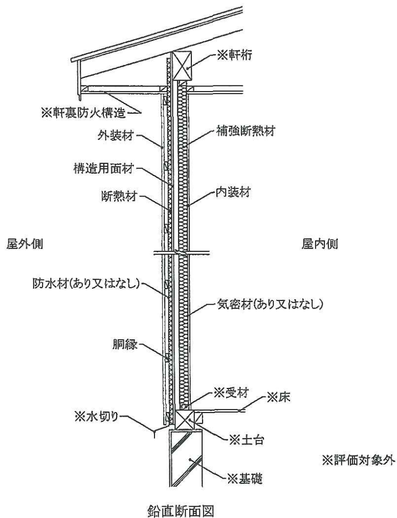
図 2 6 施工図
