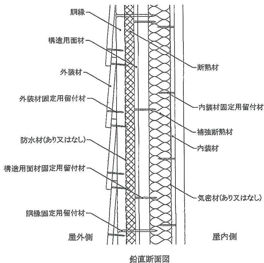
図6 構造説明図
