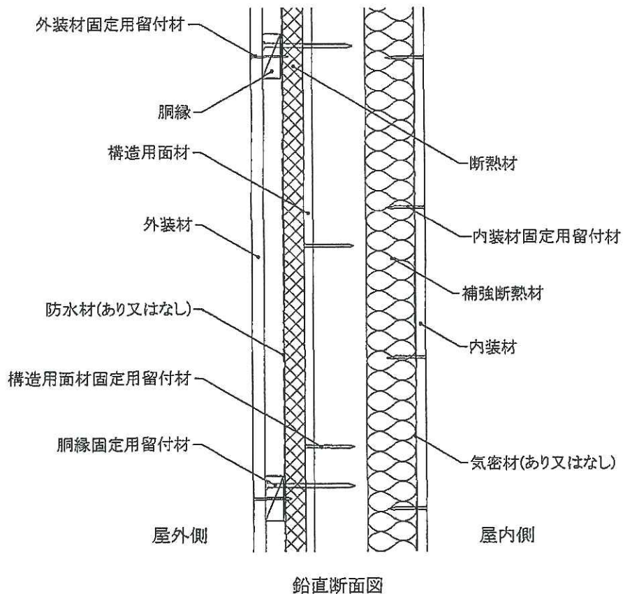
図 1 6 構造説明図
