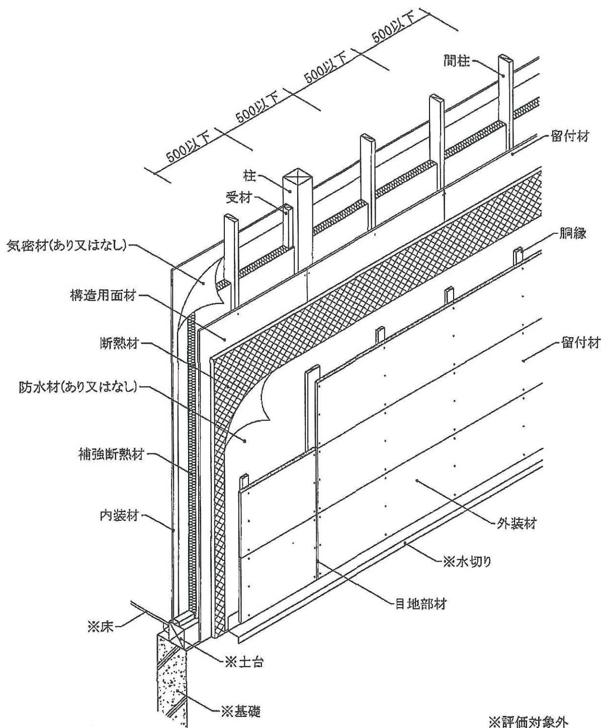
透視図
