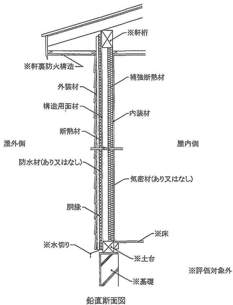
図30 施工図
