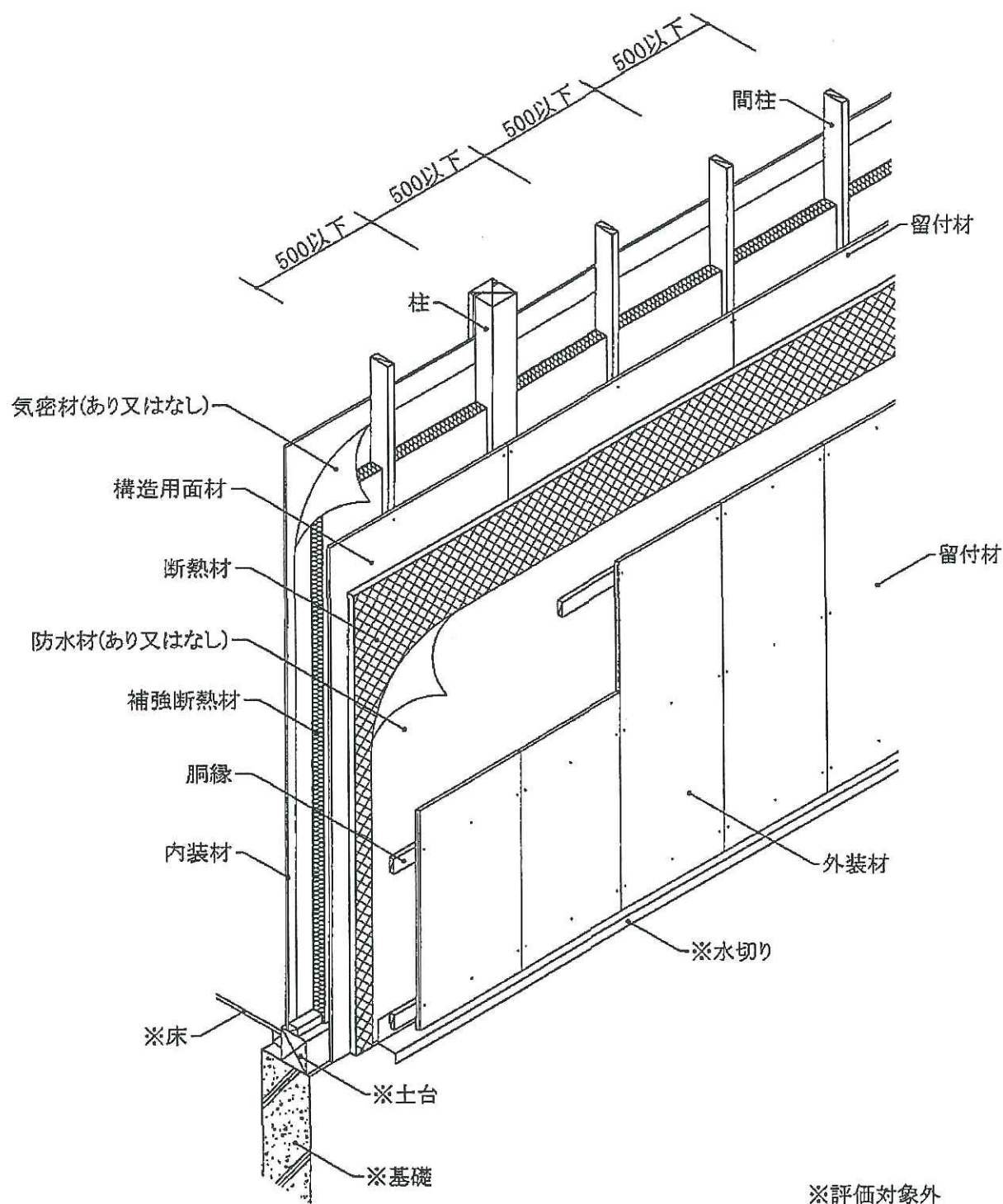
透視図
