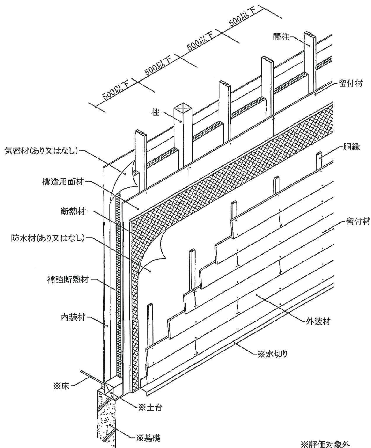
透視図
