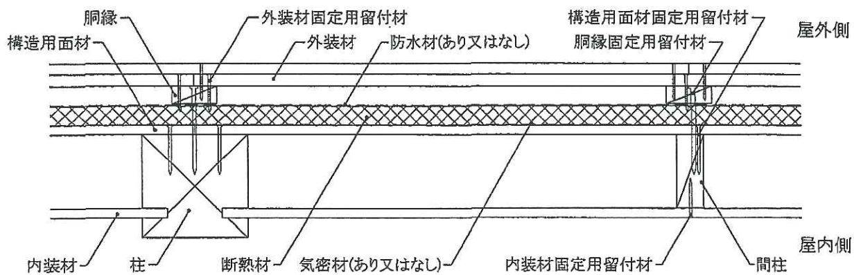
水平断面図
