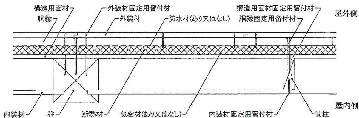
水平断面図
