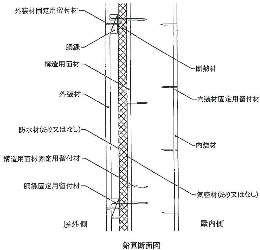
図 1 6 構造説明図
