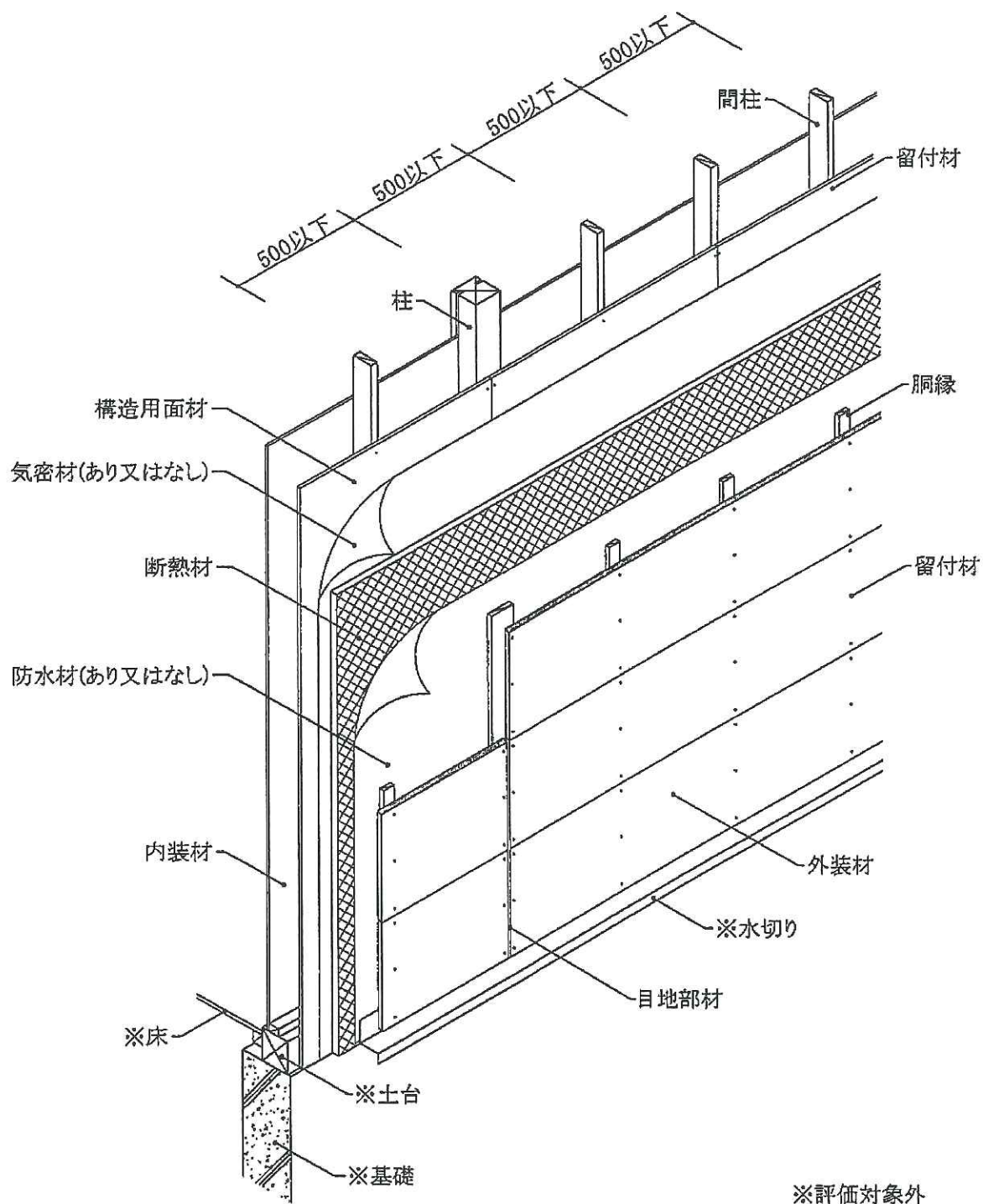
透視図
