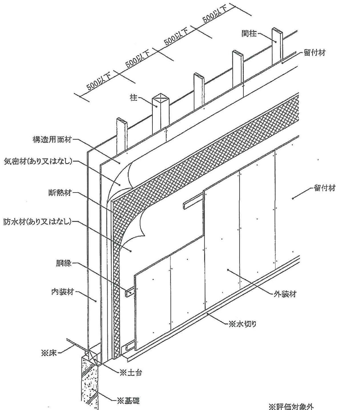
透視図
