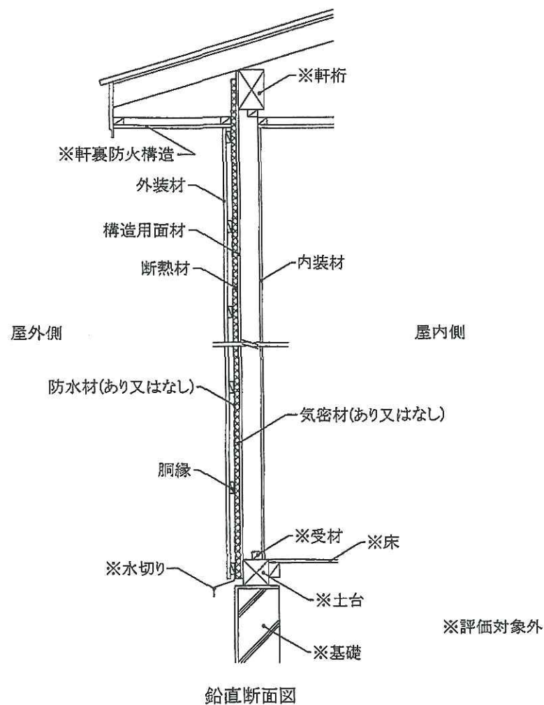
図 2 6 施工図
