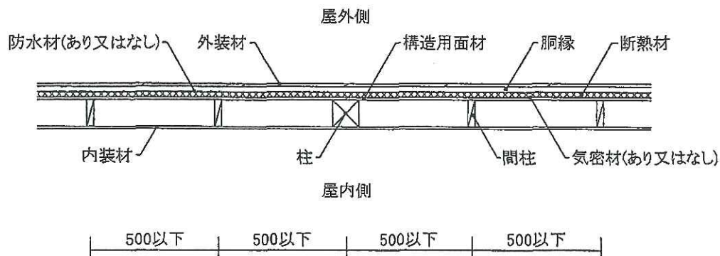
水平断面図
