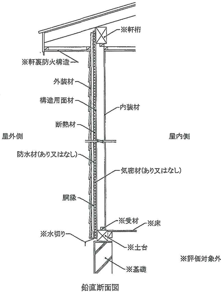
図 2 4 施工図
