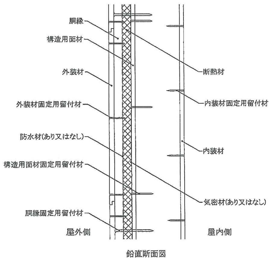
図 1 4 構造説明図
