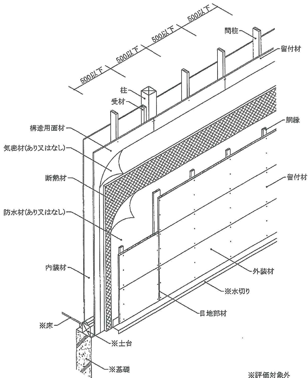
透視図
