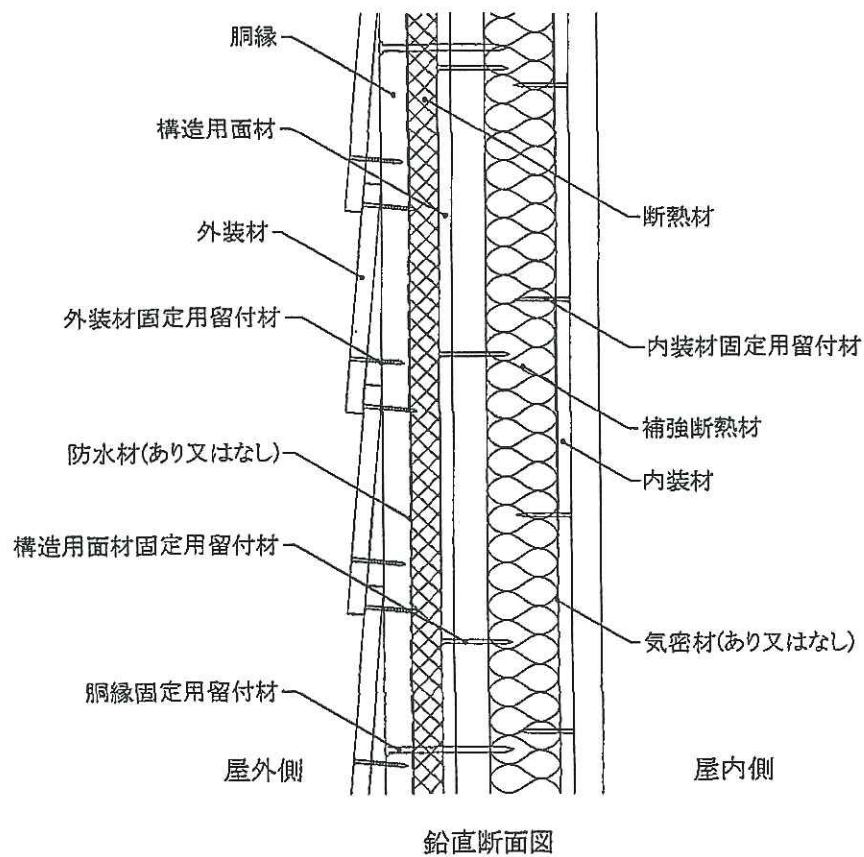
図6 構造説明図
