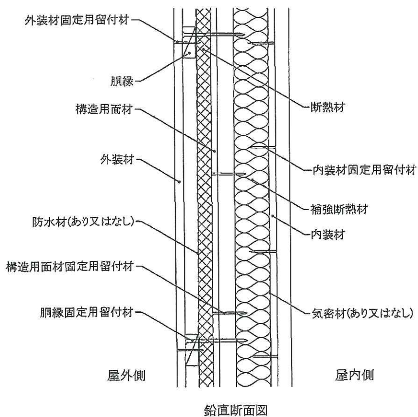
図4 構造説明図
