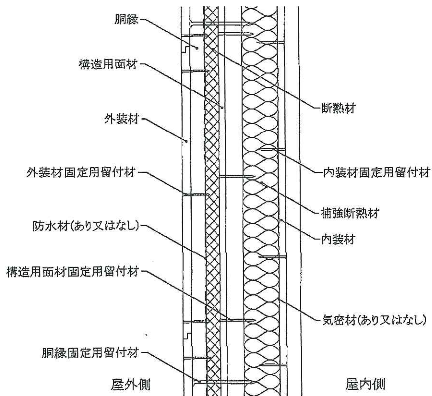
図 2 構造説明図
