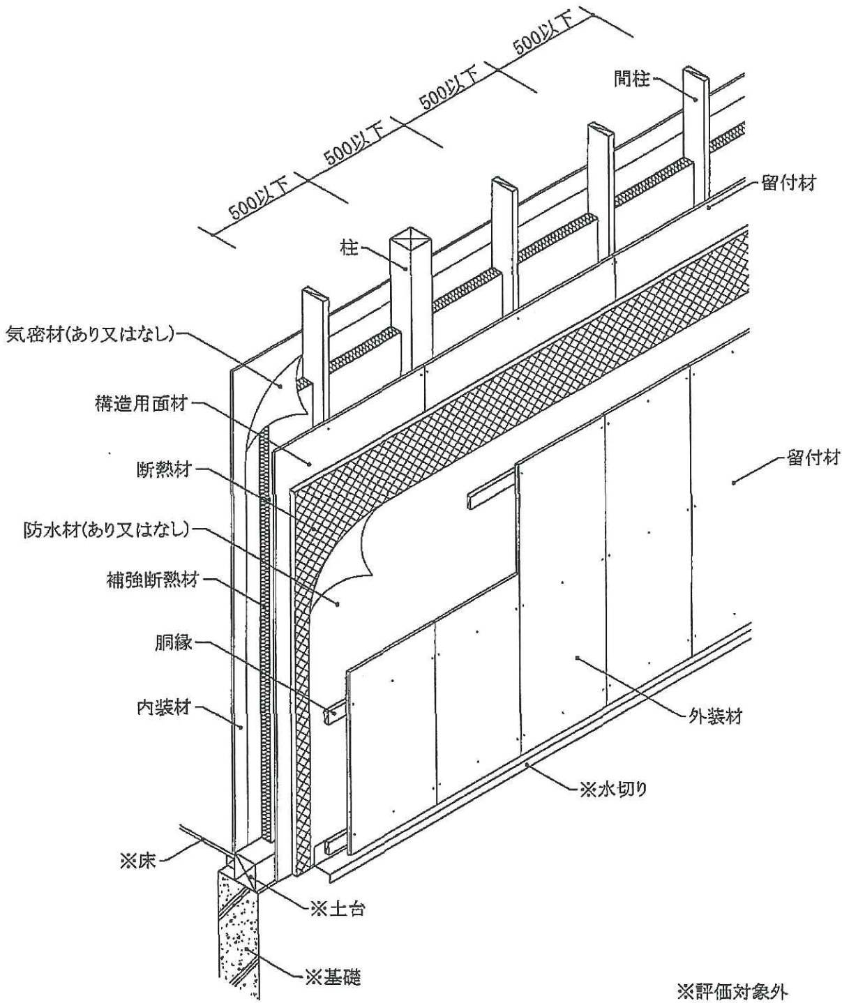
透視図
