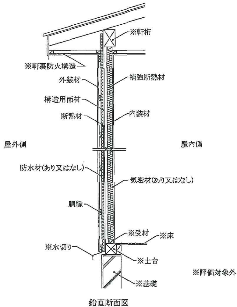
図 2 3 施工図
