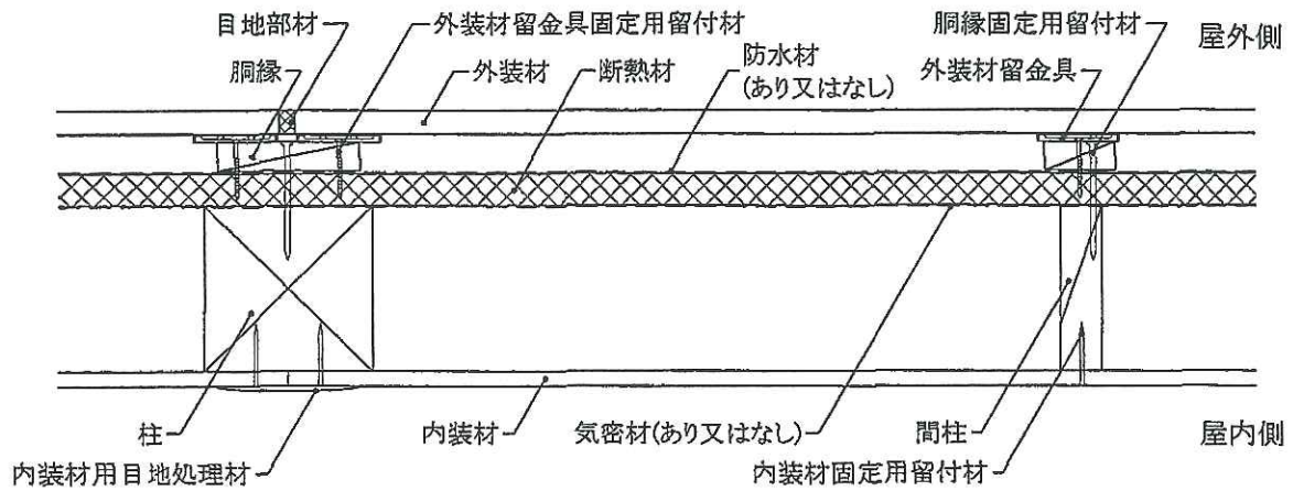
水平断面図
