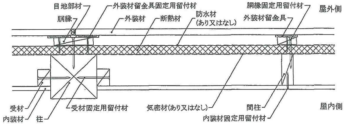
水平断面図
