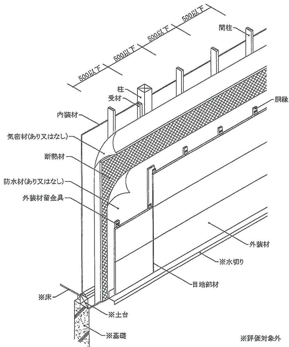
透視図
