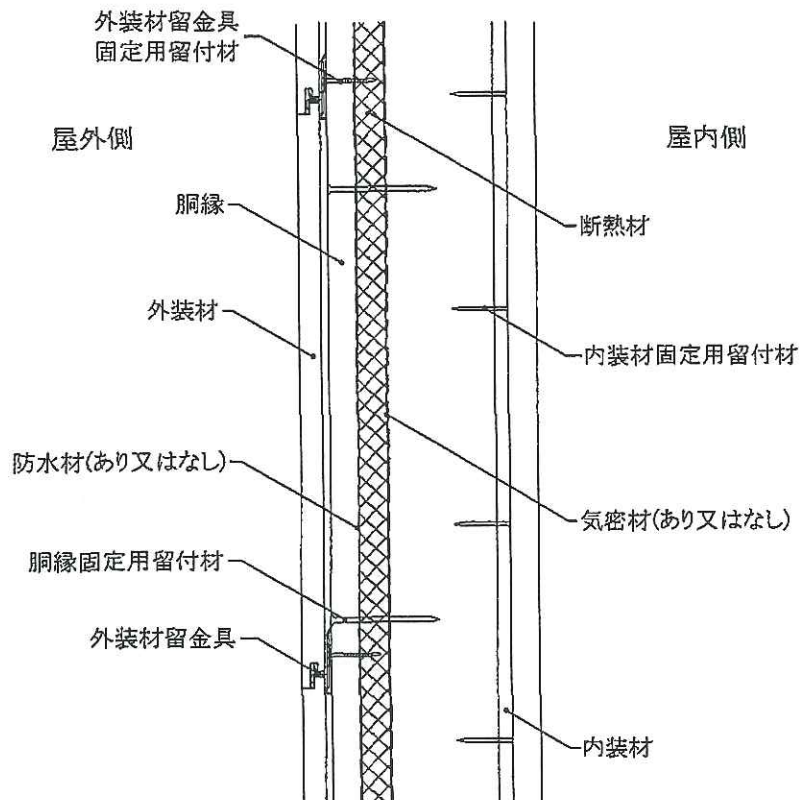
鉛直断面図
