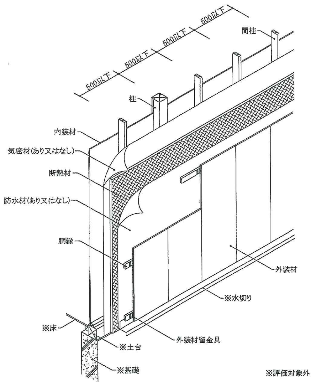
透視図
