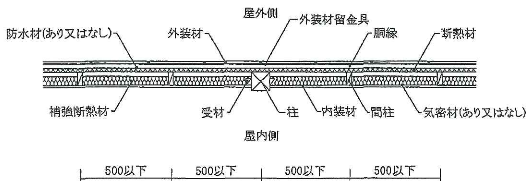
水平断面図
