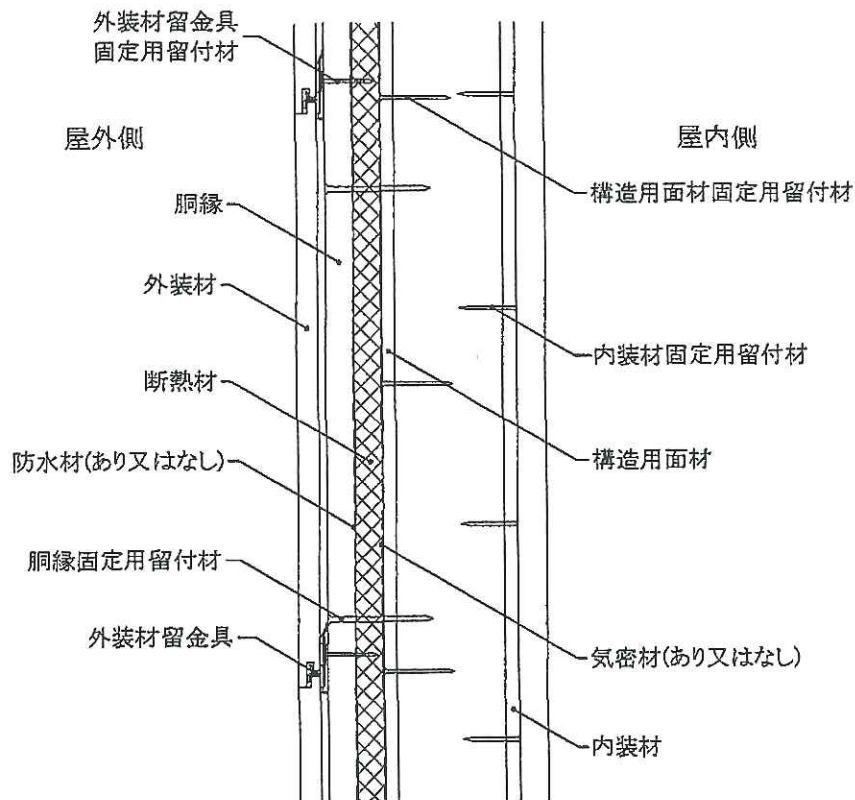
鉛直断面図
