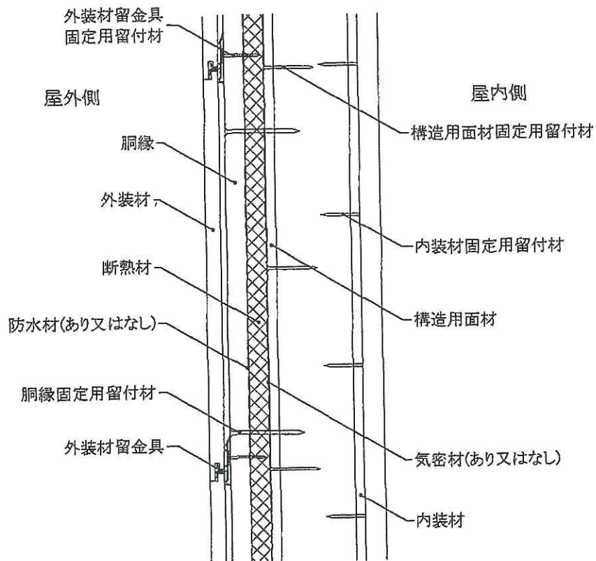
鉛直断面図
