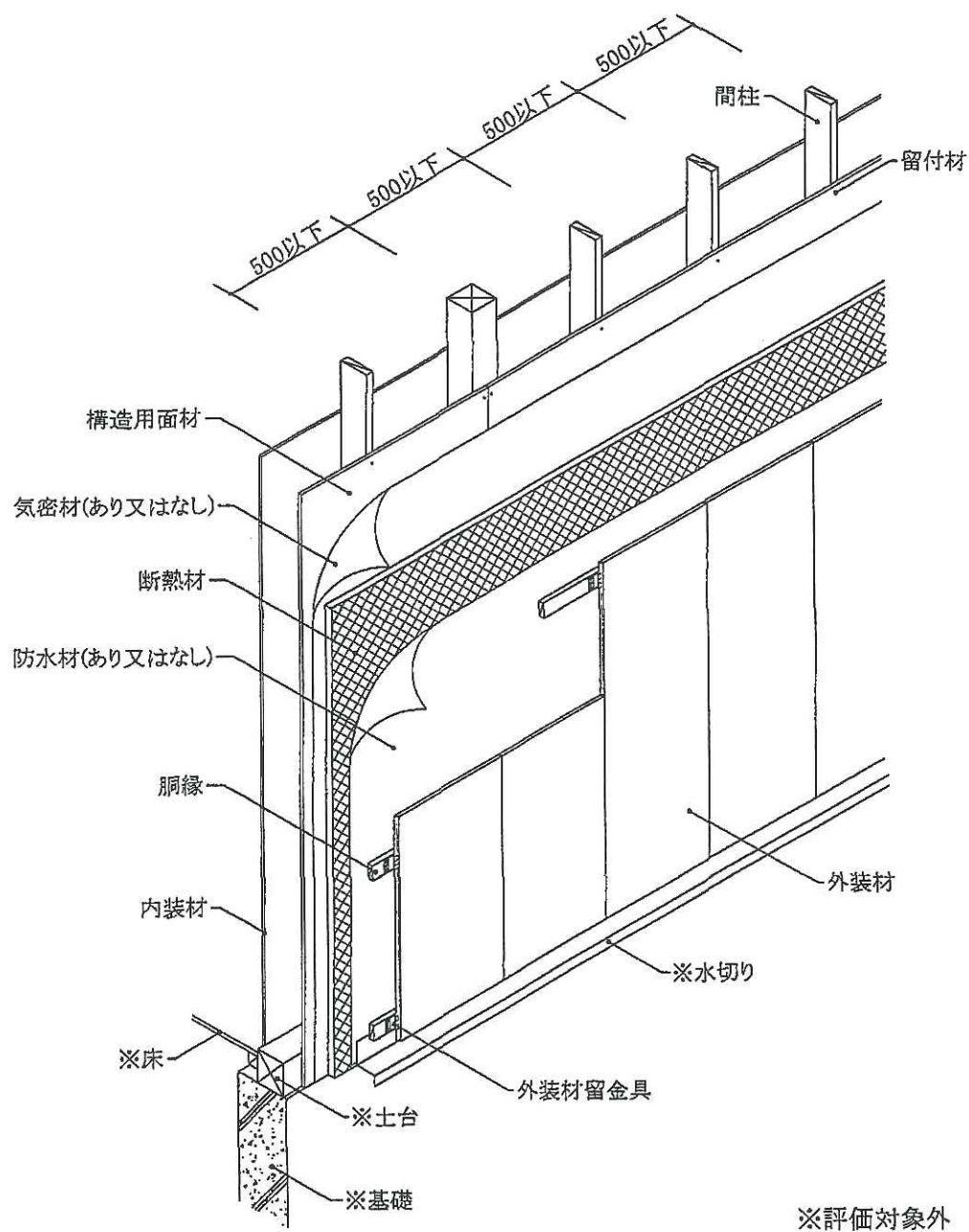
透視図
