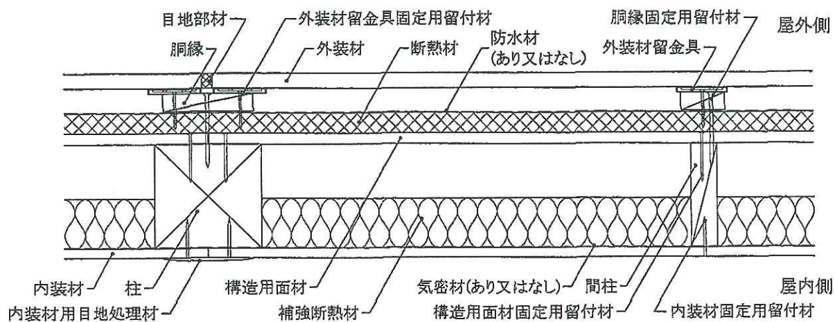
水平断面図
