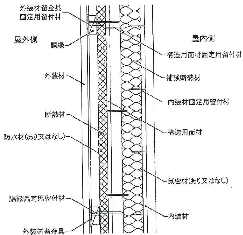
鉛直断面図
