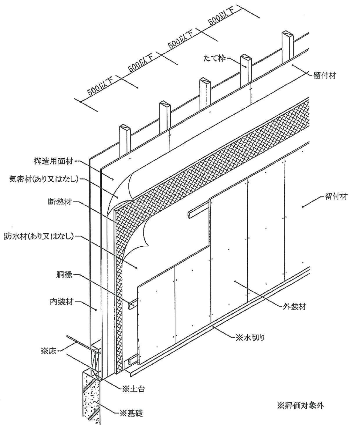
透視図
