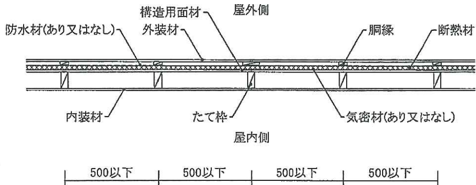
水平断面図
