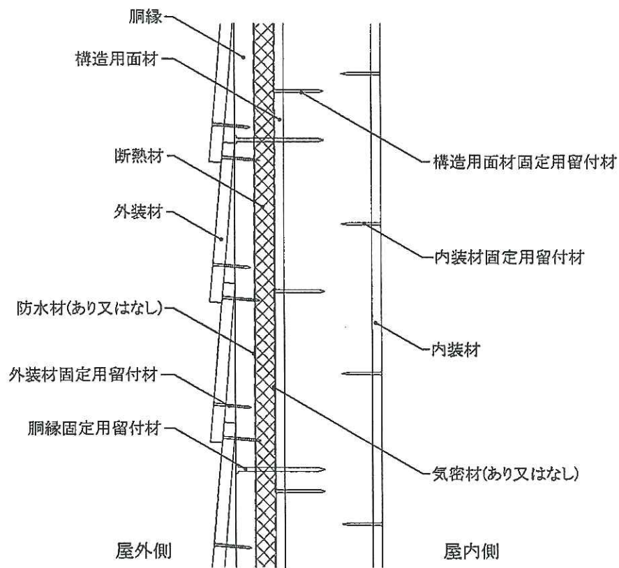
鉛直断面図
