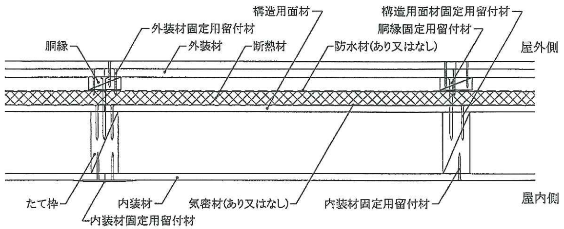
水平断面図
