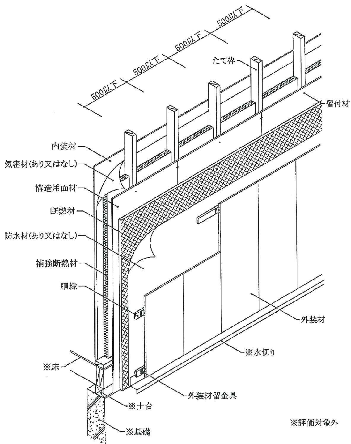
透視図
